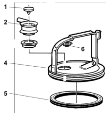
Pakningssett for spennlokk
